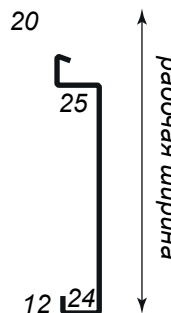
№ 6 Линеарная панель с рустом Квадро-Брус
