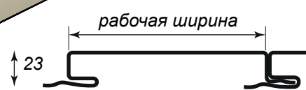
№ 4 Евробрус (Экобрус, Брус, L-брус, Сайдинг)
