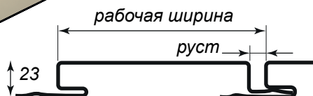
№ 3 Металлосайдинг Вагонка (L-брус)
