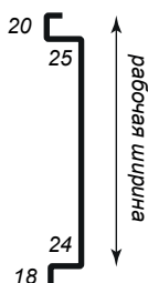
№ 5 Линеарная панель с рустом для бескаркасного строительства
